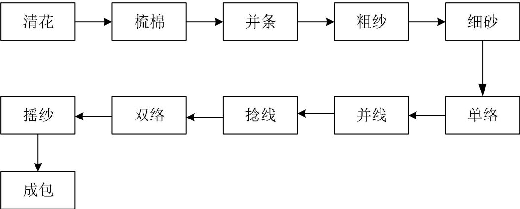
图 3 产品生产工艺流程图
